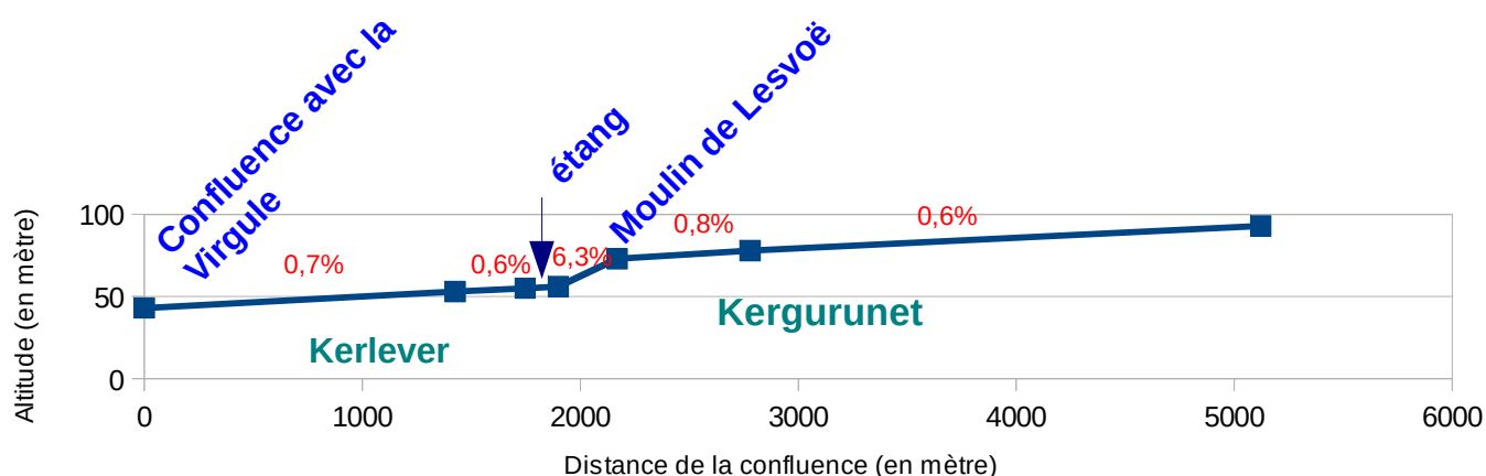
Figure 17 :Profil en long du Kerlever et du Kergurunet
