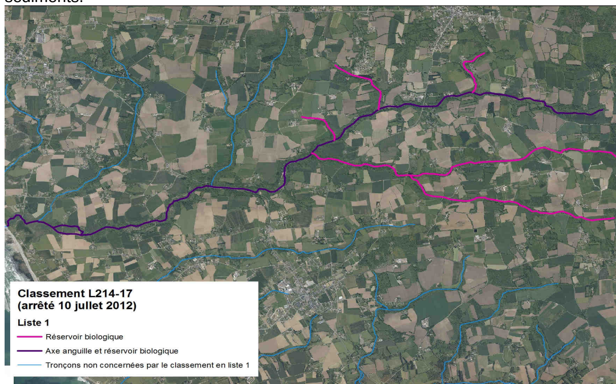
Figure 3 : Classement au titre de l'article L214-17
