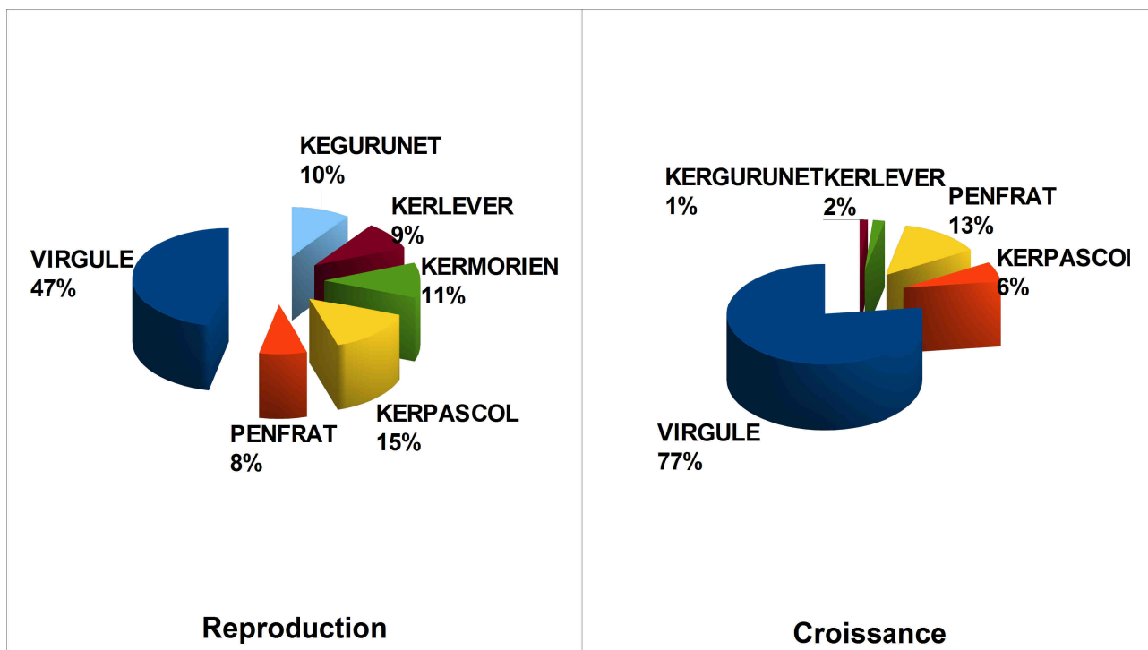
Figure 27 :Lamproie marine : répartition des surfaces de reproduction et de croissance
