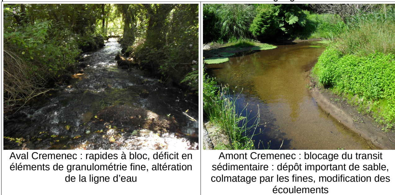
Figure 16 :Effets de l'ouvrage du moulin de Cremenec
