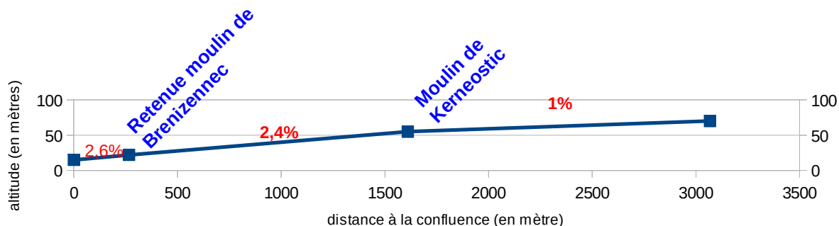
Figure 21 :Profil en long du Penfrat
