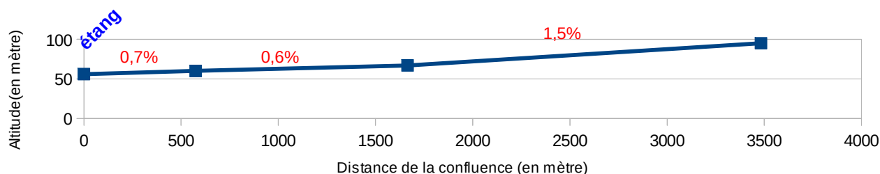
Figure 18 : Profil en long du Kermorien
