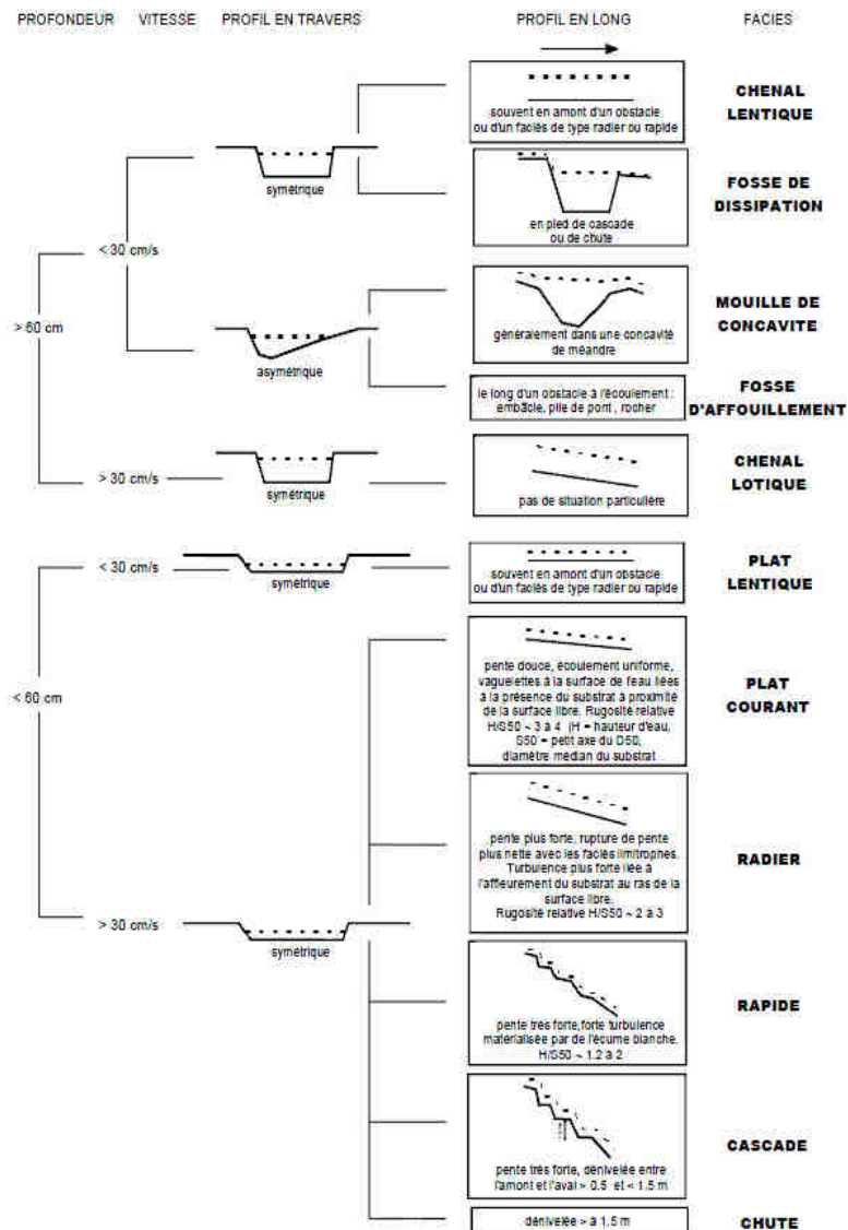
Figure 7 :Clé d'identification des faciès de Malavoi et Souchon (2003)
