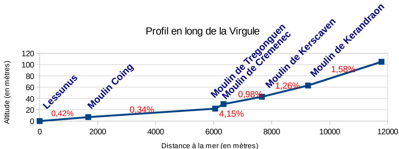
Figure 13 : profil en long du cours principal de la Virgule
