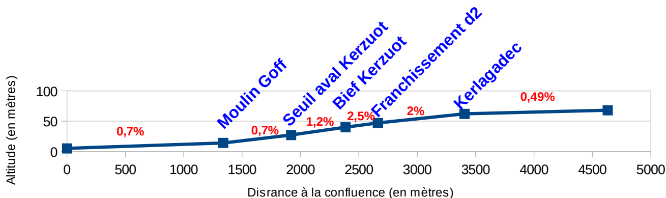
Figure 20 :Profil en long du Kerpascol
